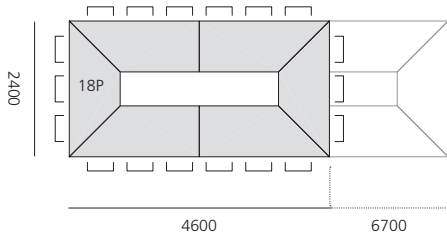
Rechteck - Ring
