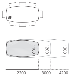
Doppel Bootform
