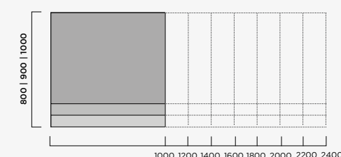
OPTIMO E23 Tischhöhe 645 mm bis 1295 mm Höhenverstellung elektrisch stufenlos Zweifaches Teleskopgestell
