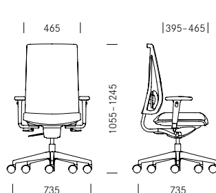
Drehstuhl, Rücken Standard Siège de bureau, dossier standard
