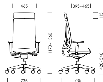
Drehstuhl, Rücken mit Aufsatz Siège de bureau, dossier avec extension
